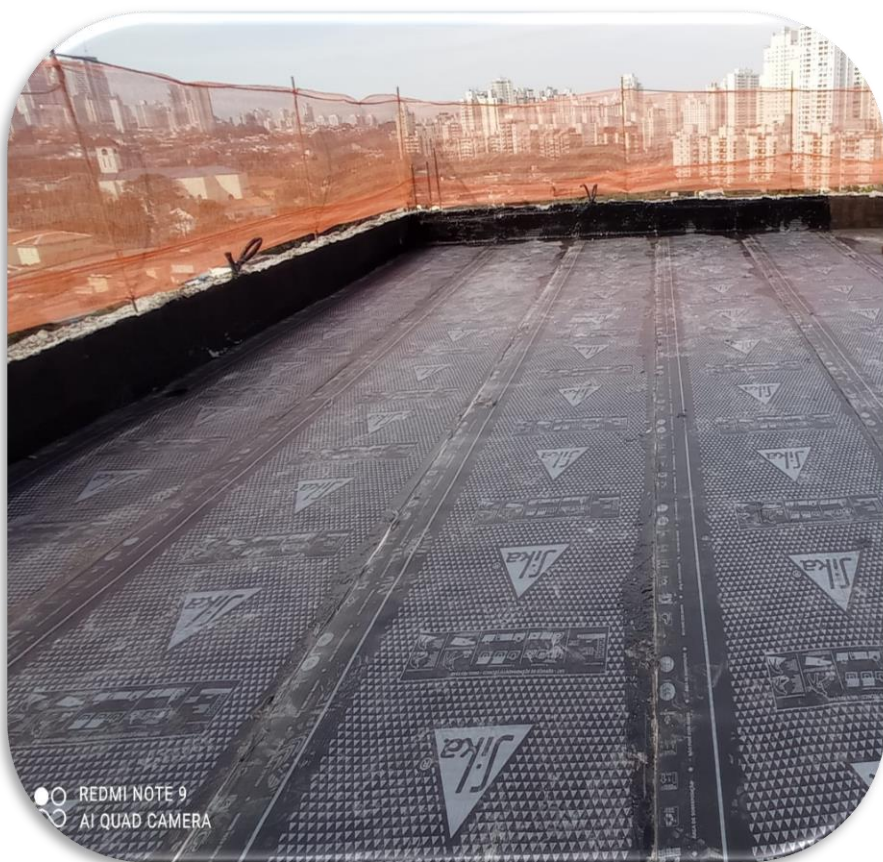
Aplicação de manta asfáltica na cobertura da torre - A
